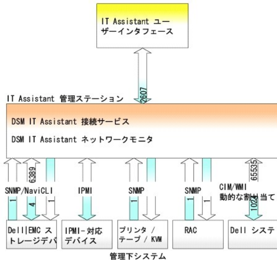
図 1-1 IT Assistant ユーザーインターフェース、サービスシステム、管理下システム
